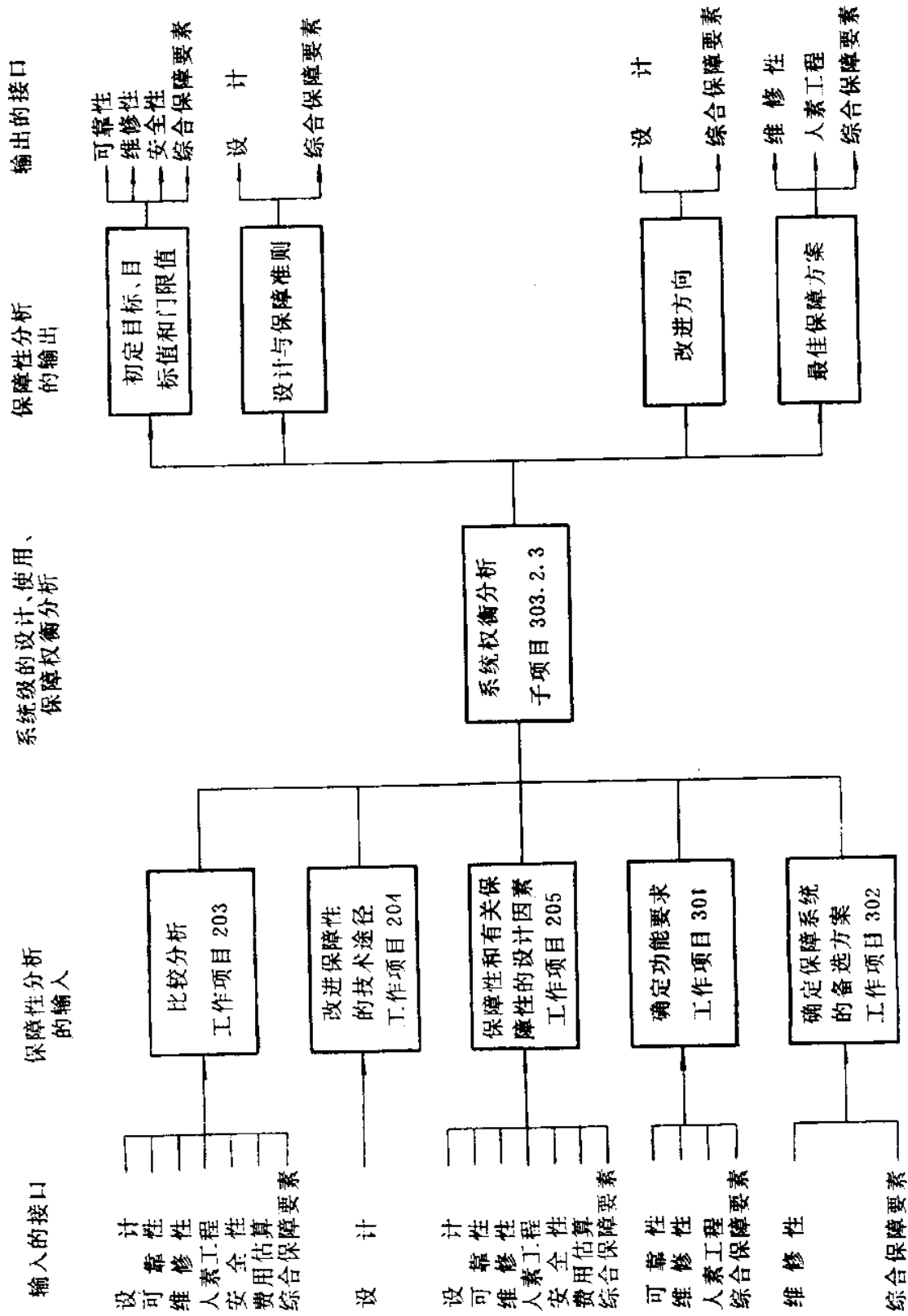
图 A1 系统级保障性分析的接口
